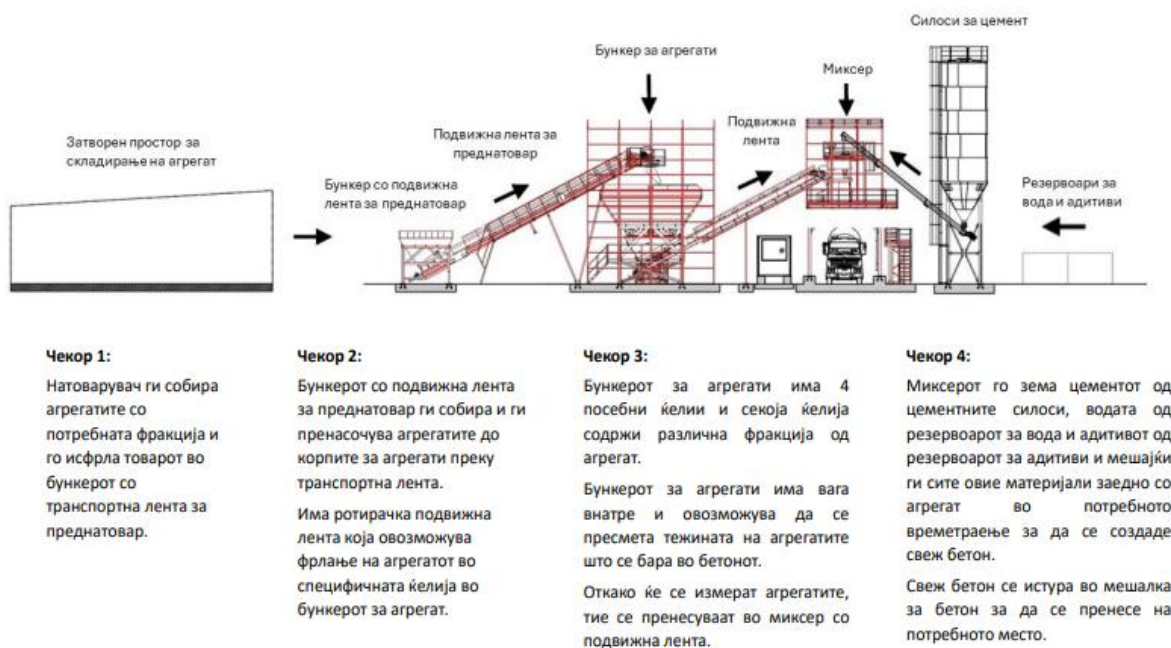
Слика бр.2 Постапка и технологија во бетонската база опишана во чекори
